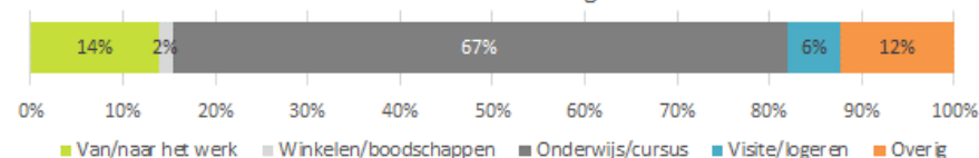
Reismotief OV-reizigers
